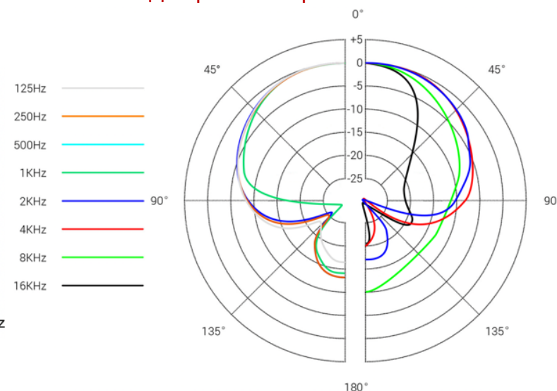
Диаграмма направленности
